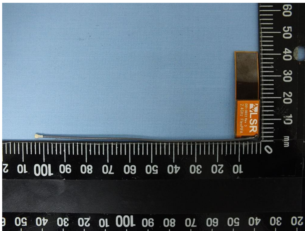
FlexPIFA antenna
