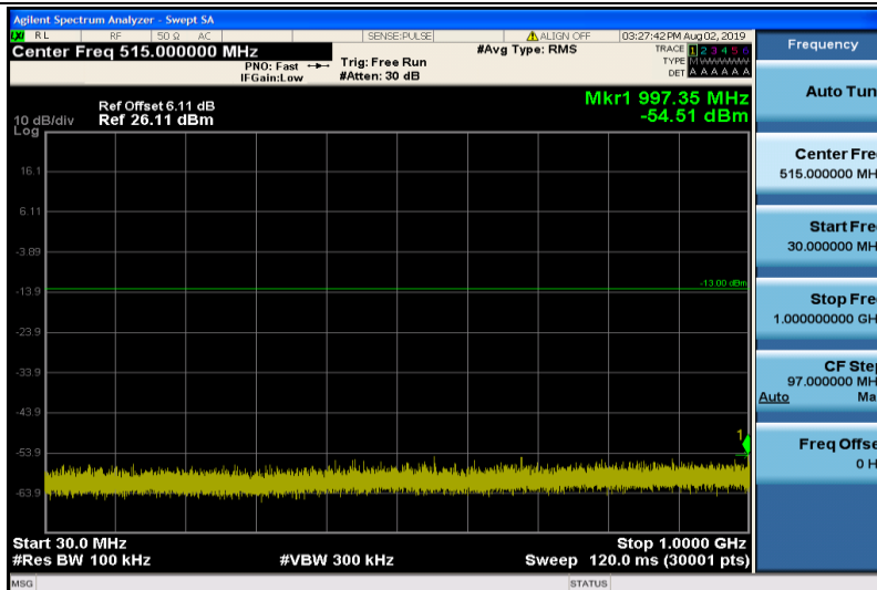
Band4-10MHz-QPSK-20000-1RB#0-30~1000MHz
