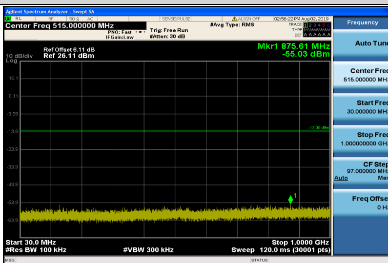
Band2-20MHz-QPSK-18900-1RB#0-30~1000MHz
