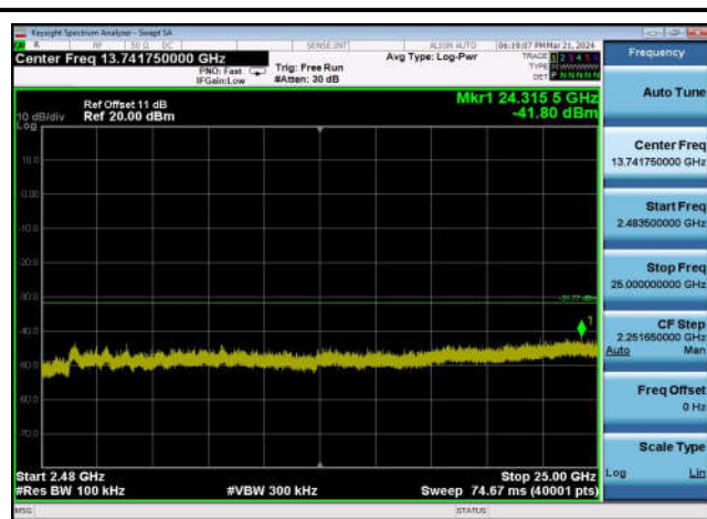
,Plot 4,2483.5MHz~25000MHz-802.11ax(4 0MHz),2437MHz,Ant1
