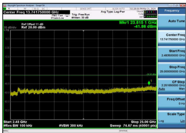
,Plot 4,2483.5MHz~25000MHz-802.11ax(4 0MHz),2452MHz,Ant0
