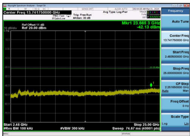
,Plot 4,2483.5MHz~25000MHz-802.11b ,2462MHz,Ant0
