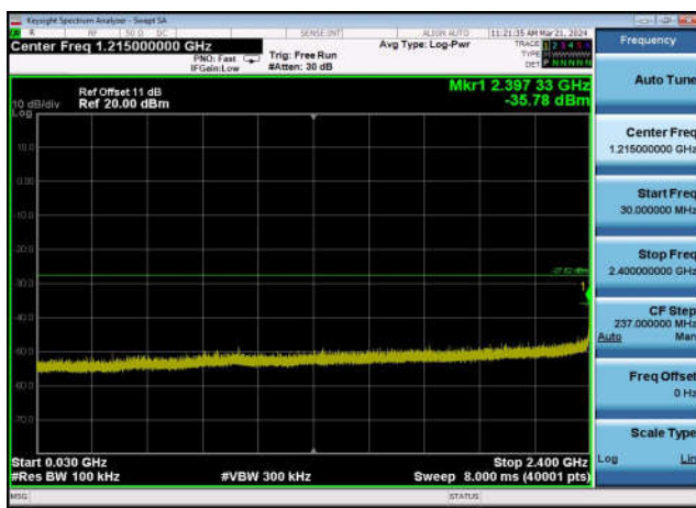
,Plot 3,30MHz~2400MHz-802.11n(20MHz) ,2437MHz,Ant0
