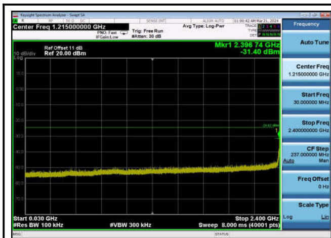
,Plot 3,30MHz~2400MHz-802.11g,2437MHz ,Ant0
