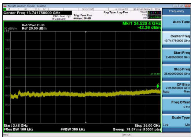
,Plot 4,2483.5MHz~25000MHz-802.11ax(4 0MHz),2422MHz,Ant0
