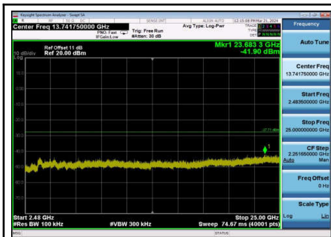
,Plot 4,2483.5MHz~25000MHz-802.11ax(2 0MHz),2437MHz,Ant0
