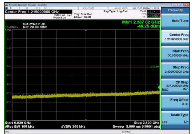
,Plot 3,30MHz~2400MHz-802.11b,2462MHz ,Ant1
