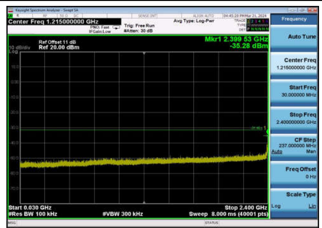
,Plot 3,30MHz~2400MHz-802.11n(40MHz) ,2437MHz,Ant1
