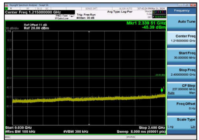
,Plot 3,30MHz~2400MHz-802.11n(20MHz) ,2462MHz,Ant1
