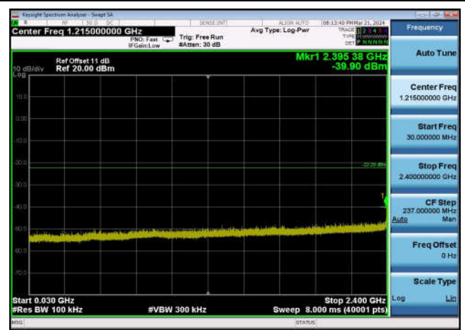
,Plot 3,30MHz~2400MHz-802.11b,2437MHz ,Ant1
