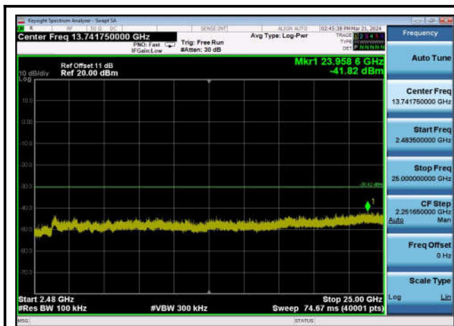
,Plot 4,2483.5MHz~25000MHz-802.11ax(4 0MHz),2437MHz,Ant0
