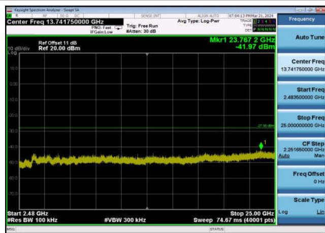
,Plot 4,2483.5MHz~25000MHz-802.11ax(4 0MHz),2422MHz,Ant1
