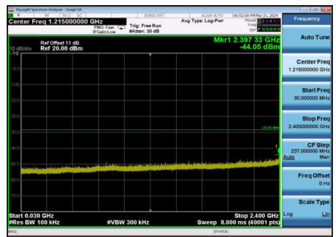
,Plot 3,30MHz~2400MHz-802.11ax(20MHz) ,2437MHz,Ant1
