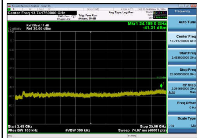
,Plot 4,2483.5MHz~25000MHz-802.11ax(4 0MHz),2452MHz,Ant0
