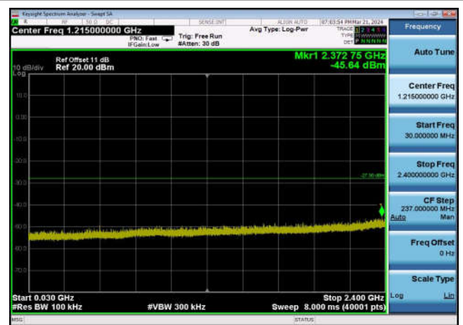
,Plot 3,30MHz~2400MHz-802.11ax(40MHz) ,2422MHz,Ant1
