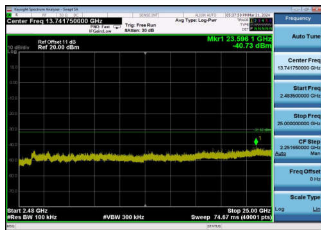
,Plot 4,2483.5MHz~25000MHz-802.11ax(4 0MHz),2452MHz,Ant1
