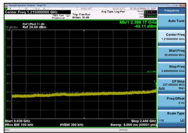
,Plot 3,30MHz~2400MHz-802.11n(20MHz) ,2437MHz,Ant1
