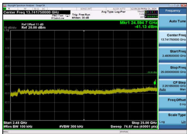
,Plot 4,2483.5MHz~25000MHz-802.11ax(2 0MHz),2462MHz,Ant0
