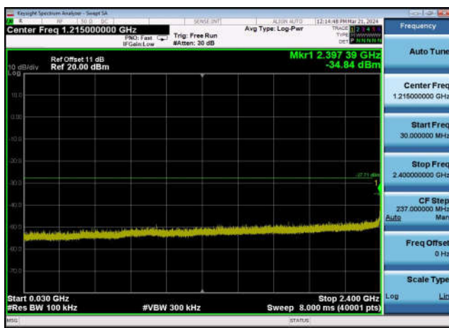
,Plot 3,30MHz~2400MHz-802.11ax(20MHz) ,2437MHz,Ant0
