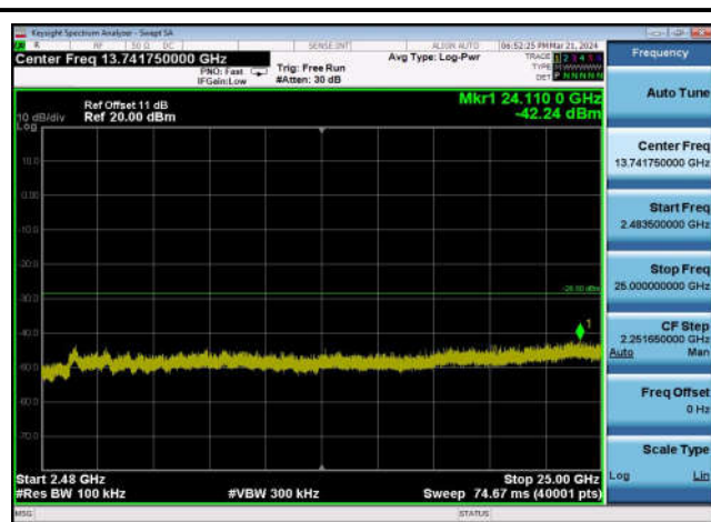
,Plot 4,2483.5MHz~25000MHz-802.11ax(2 0MHz),2437MHz,Ant1
