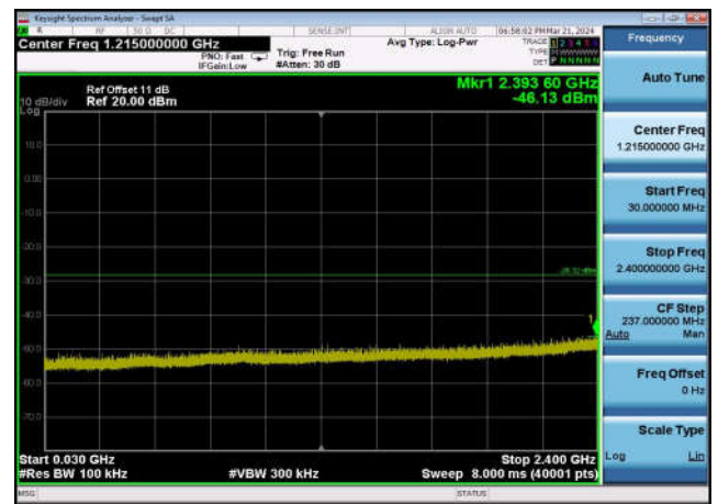
,Plot 3,30MHz~2400MHz-802.11ax(20MHz) ,2462MHz,Ant1
