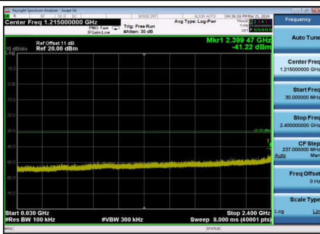
,Plot 3,30MHz~2400MHz-802.11n(40MHz) ,2437MHz,Ant0
