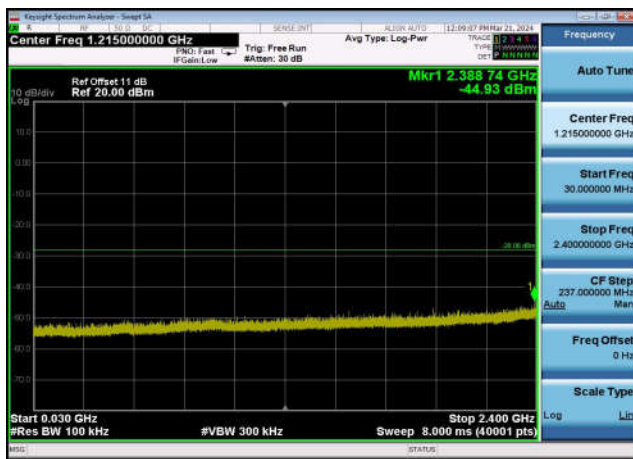
,Plot 3,30MHz~2400MHz-802.11ax(20MHz) ,2462MHz,Ant0
