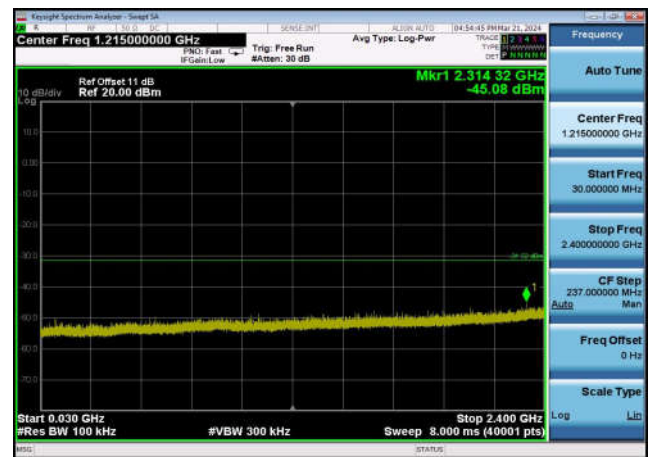
,Plot 3,30MHz~2400MHz-802.11n(40MHz) ,2452MHz,Ant1
