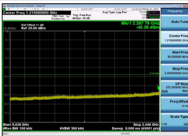
,Plot 3,30MHz~2400MHz-802.11ax(40MHz) ,2422MHz,Ant0
