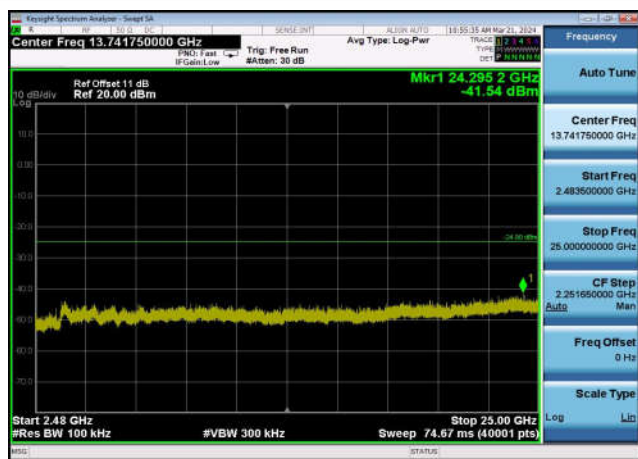
,Plot 4,2483.5MHz~25000MHz-802.11g ,2462MHz,Ant0
