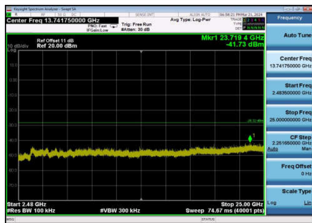
,Plot 4,2483.5MHz~25000MHz-802.11ax(2 0MHz),2462MHz,Ant1
