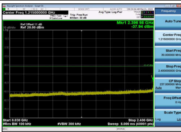
,Plot 3,30MHz~2400MHz-802.11b,2437MHz ,Ant0
