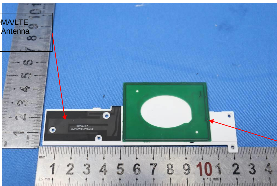
NFC Antenna
