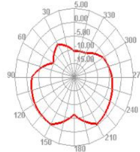
2450.000MHz E2
