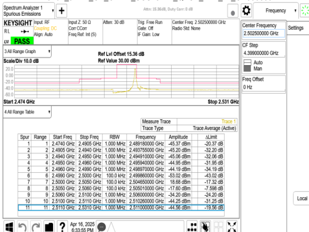
Band7_5MHz_CP_OFDM_SCS15kHz_QPSK_RB1_24_CH500500
