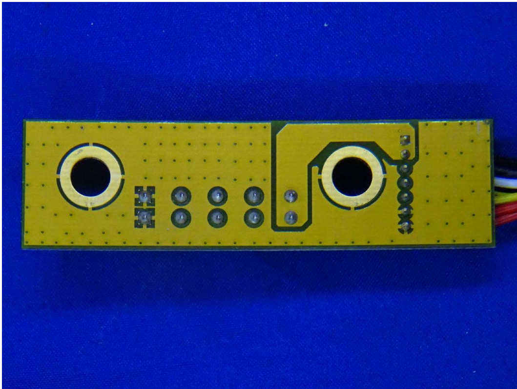
(192) EUT Photo
