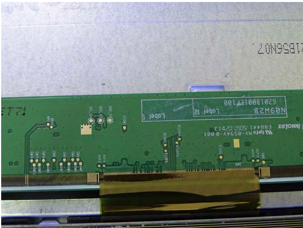
(209) EUT Photo
