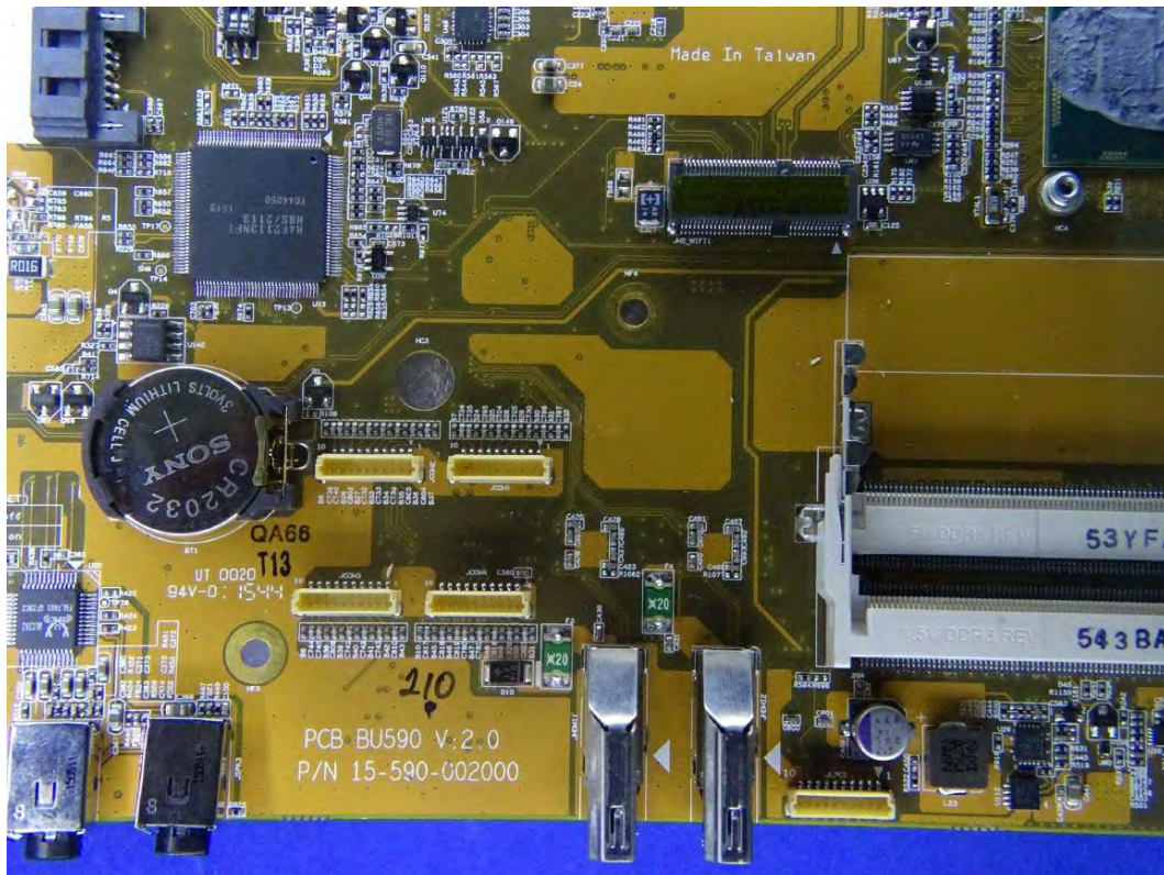
(182) EUT Photo
