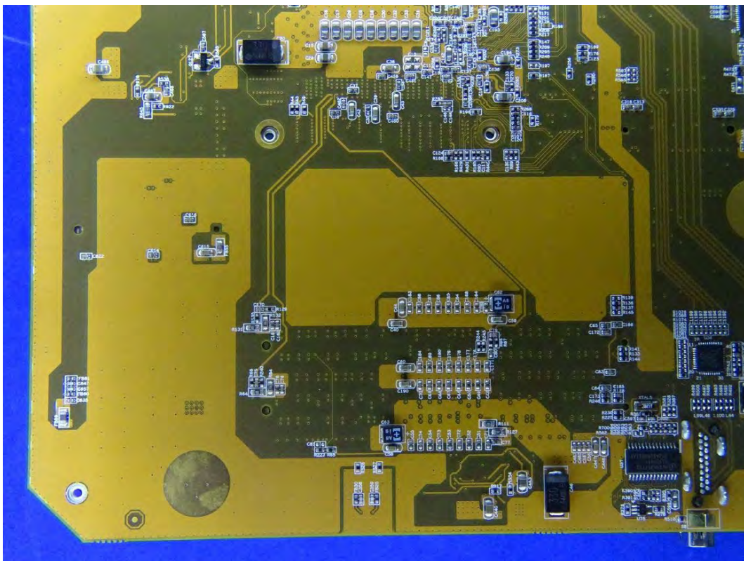
(187) EUT Photo
