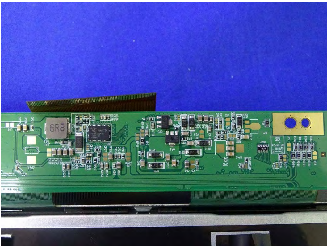
(205) EUT Photo
