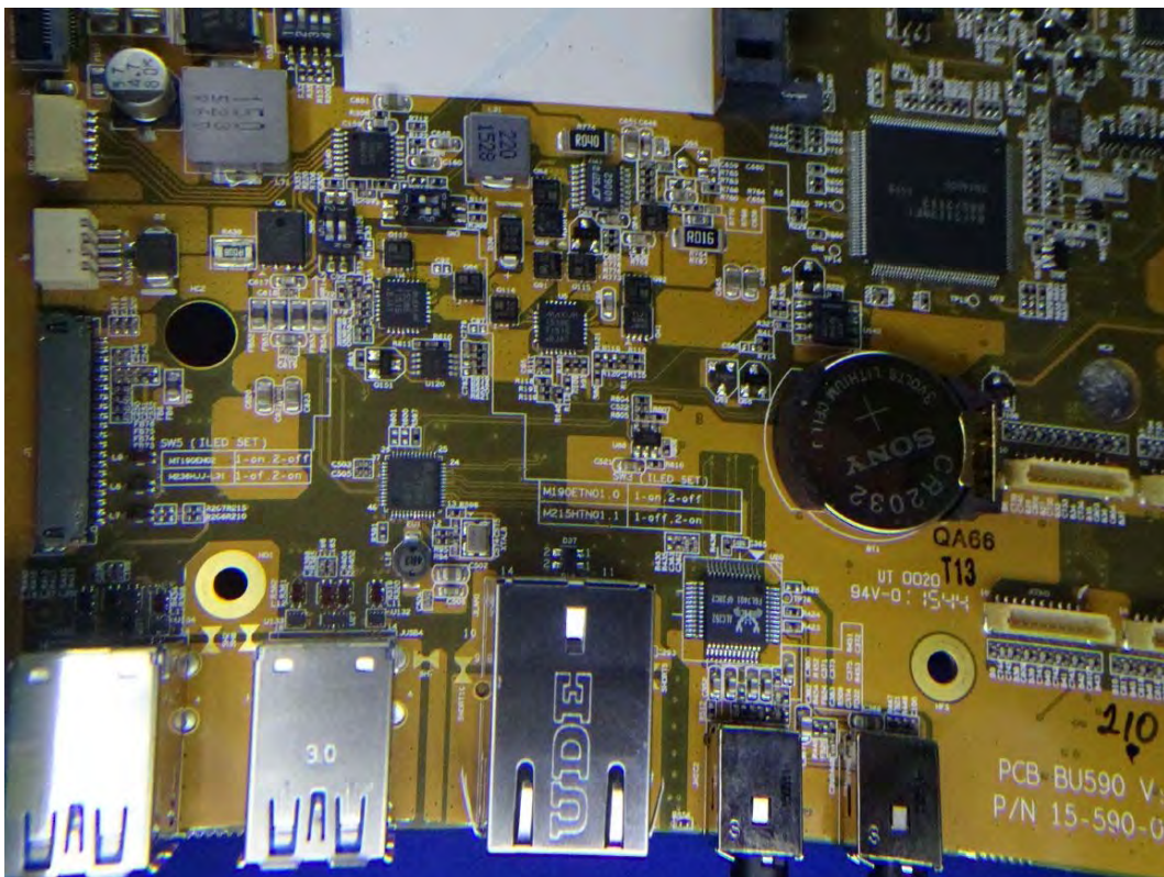
(181) EUT Photo
