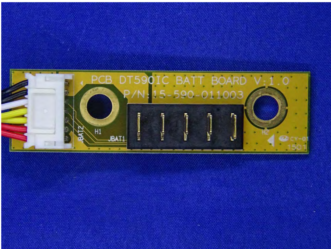
(191) EUT Photo
