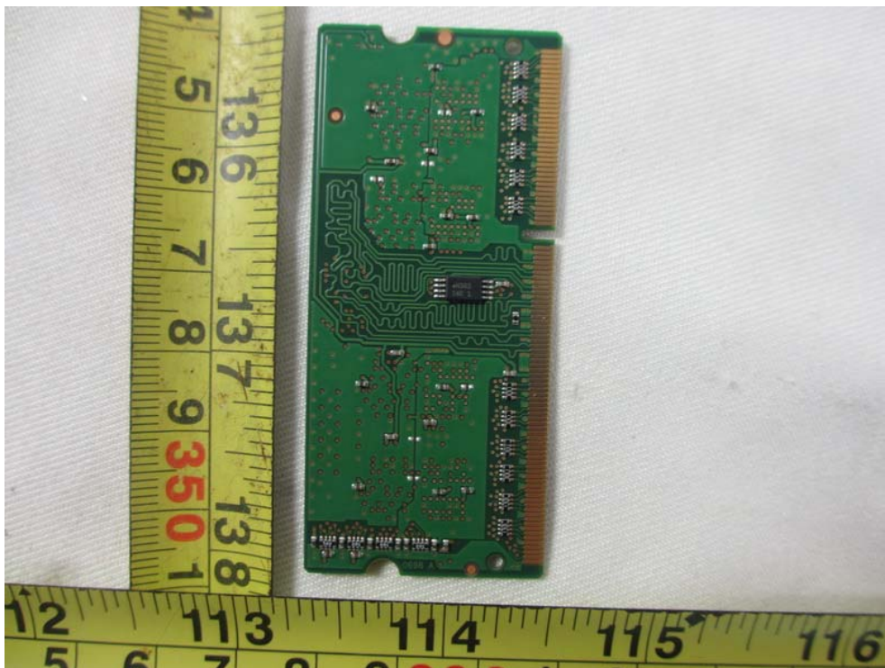
Main module
