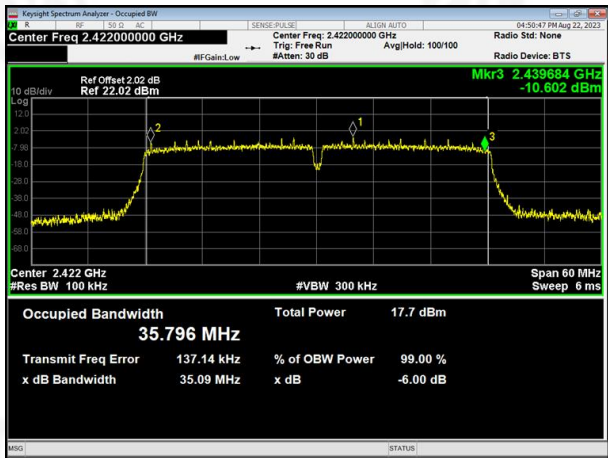
802.11ax(HE40)
