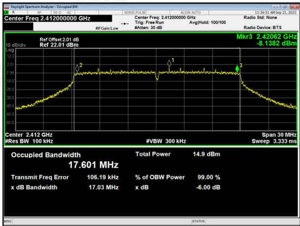
802.11ax(HE20)
