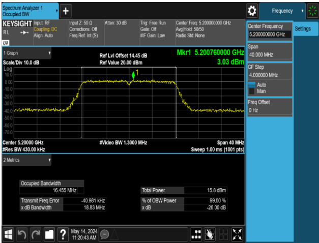
11A-Ant1-5200
