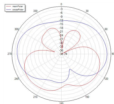
Theta=90 freq=2400MHz
