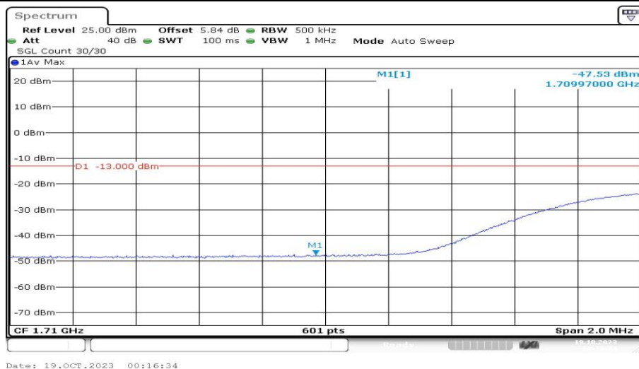
Band4-20MHz-QPSK-20050-1RB#99-PASS
