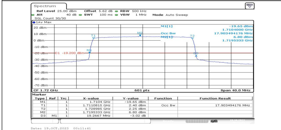
Band4-20MHz-QPSK-20050-100RB#0-PASS
