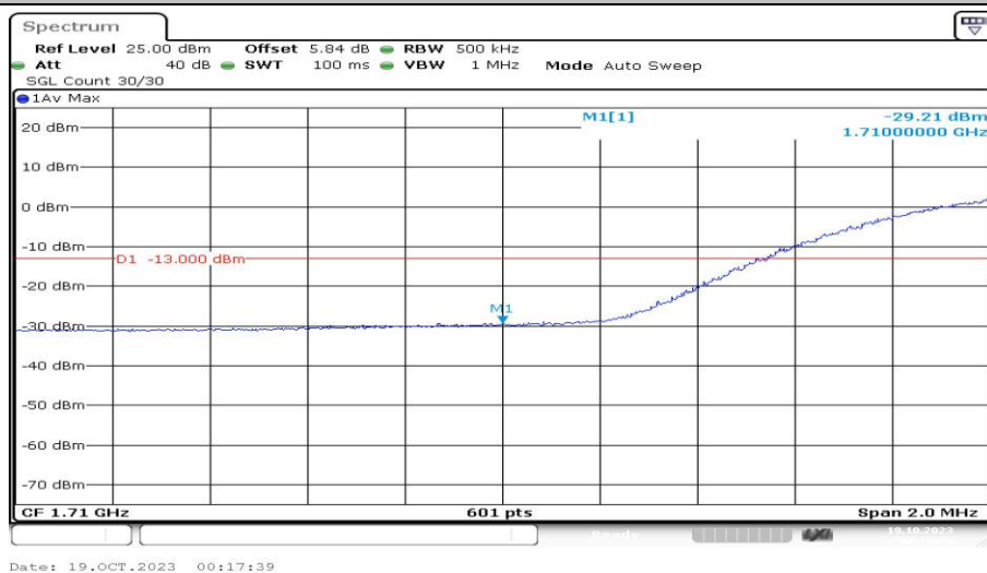
Band4-20MHz-QPSK-20050-100RB#0-PASS
