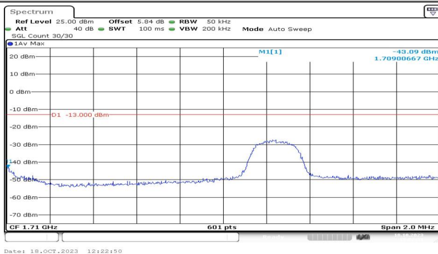
Band4-3MHz-QPSK-19965-1RB#14-PASS
