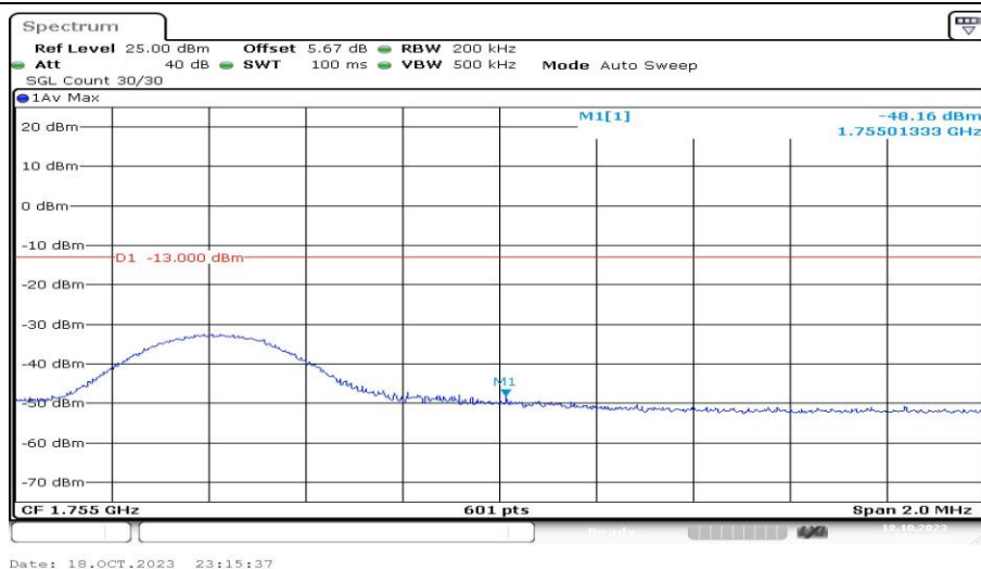
Band4-10MHz-QPSK-20350-1RB#0-PASS
