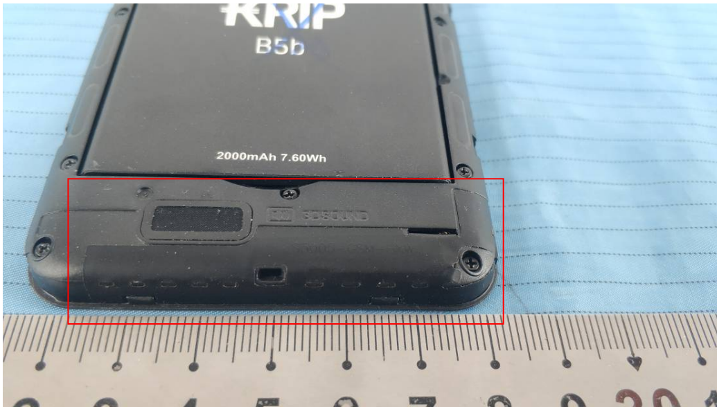
GSM&WCDMA Antenna
