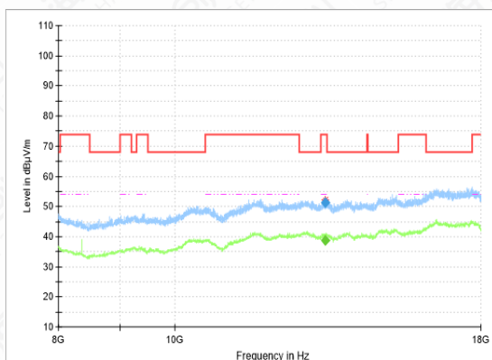
RSE-11AC(40M)-CH151-8GHz-18GHz
