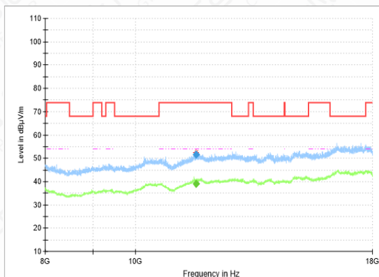
RSE-11N-CH157-8GHz-18GHz
