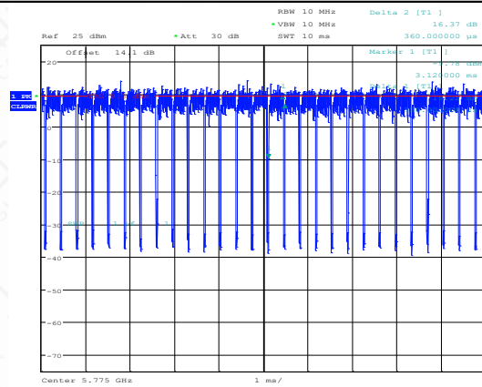
NTNV-11AC80SISO-Ant1-5775
