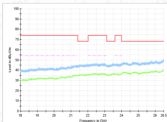
RSE-11AC(40M)-CH151-18GHz-26.5GHz
