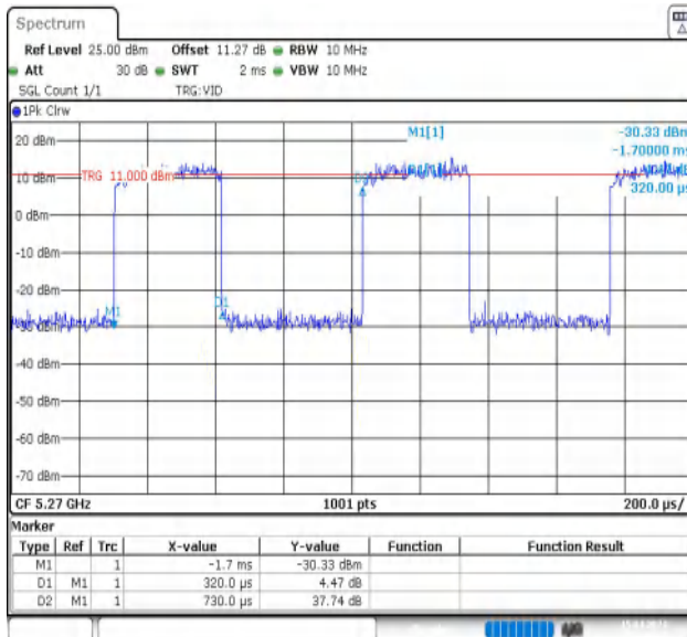
NTNV-11N40MIMO-Ant1-5270
