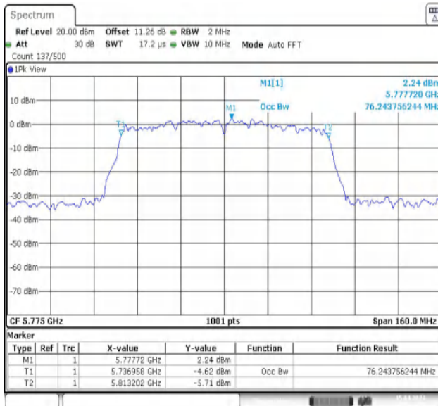
11AC80MIMO-Ant1-5775
