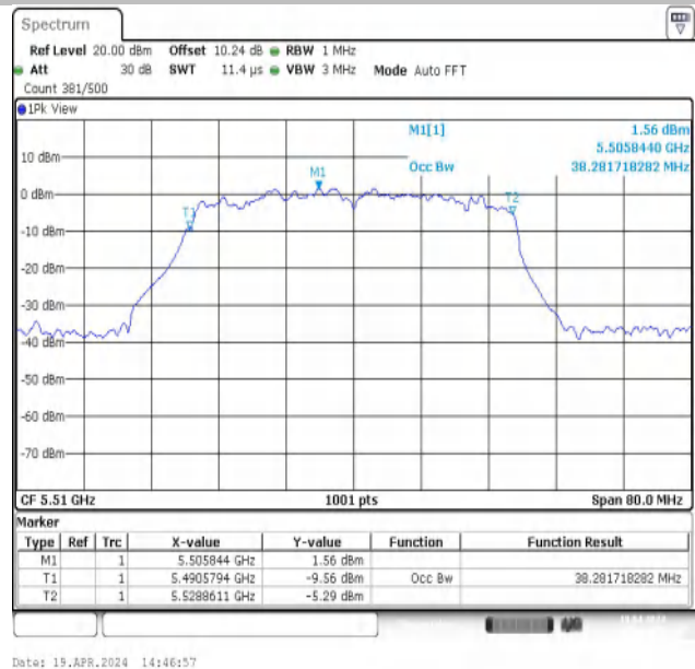
11AX40MIMO-Ant2-5510
