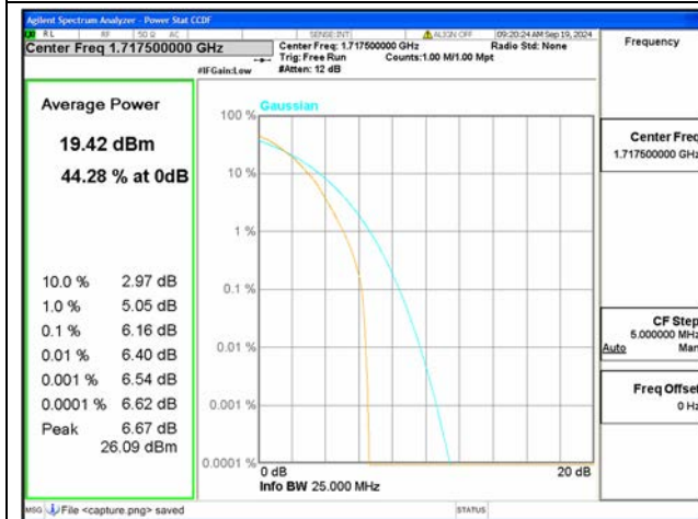
B66 / 15MHz / Low CH / 64QAM
