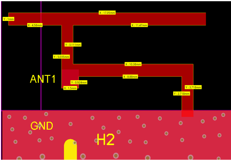
天线尺寸/ANT Size
