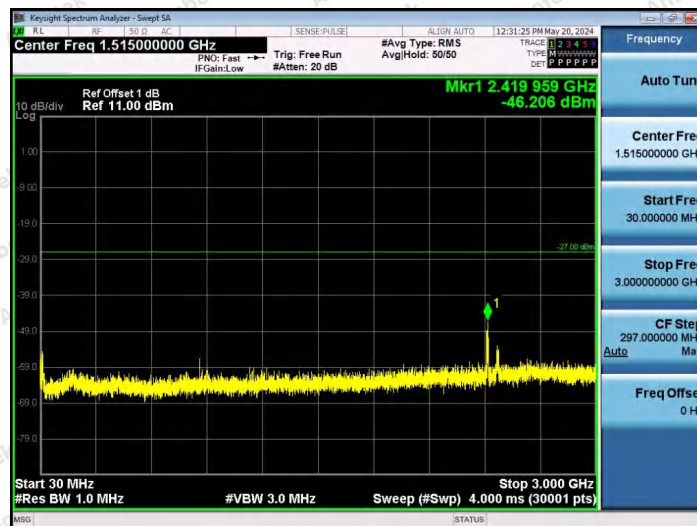
11AX80SISO-Ant1-6145-106Tone-RU53-30~3000-PASS
