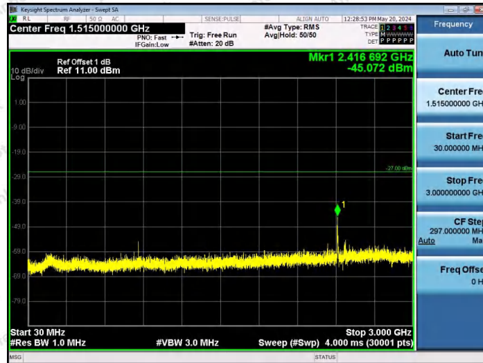
11AX80SISO-Ant1-6145-52Tone-RU52-30~3000-PASS
