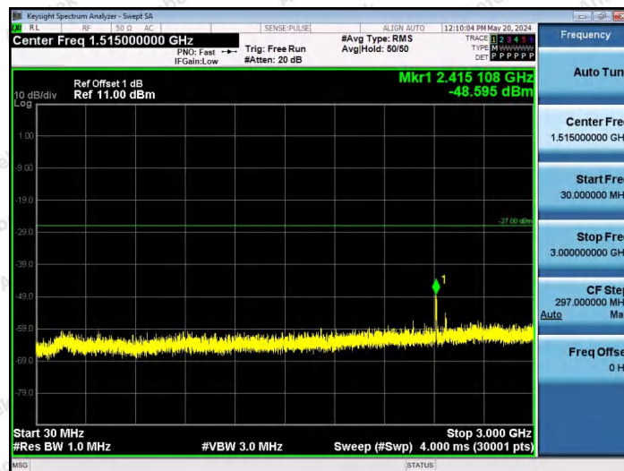
11AX80SISO-Ant1-5985-242Tone-RU64-30~3000-PASS
