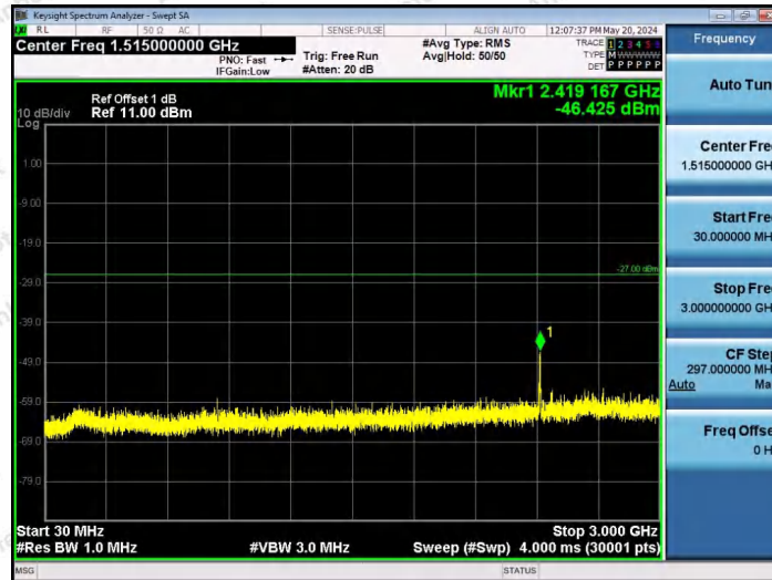
11AX80SISO-Ant1-5985-242Tone-RU61-30~3000-PASS
