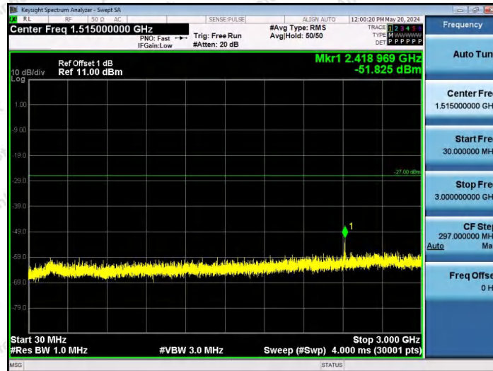
11AX80SISO-Ant1-5985-52Tone-RU52-30~3000-PASS
