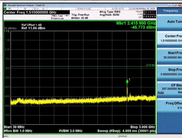
11AX80SISO-Ant1-6145-52Tone-RU37-30~3000-PASS
