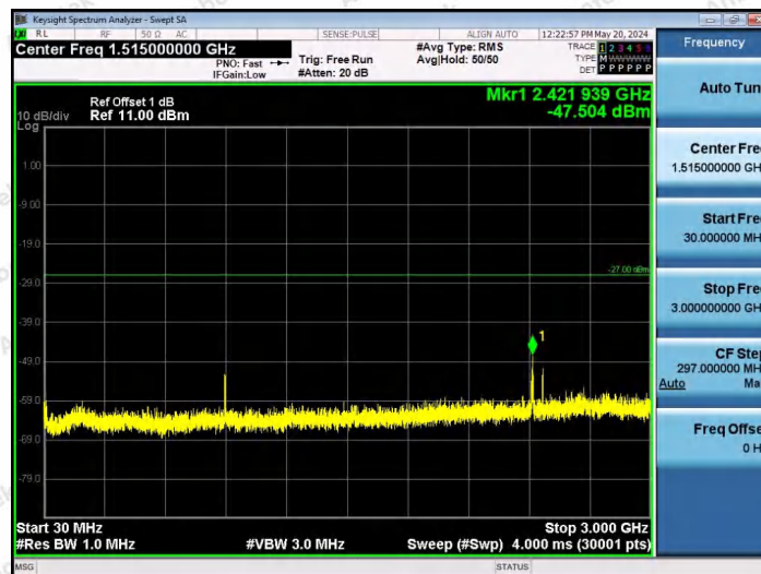
11AX80SISO-Ant1-6145-26Tone-RU36-30~3000-PASS
