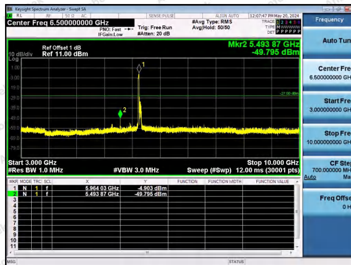
11AX80SISO-Ant1-5985-242Tone-RU61-3000~10000-PASS
