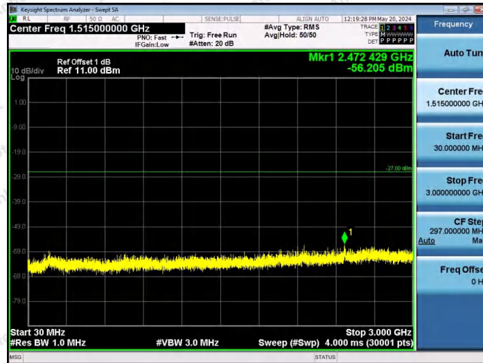
11AX80SISO-Ant1-6145-26Tone-RU0-30~3000-PASS
