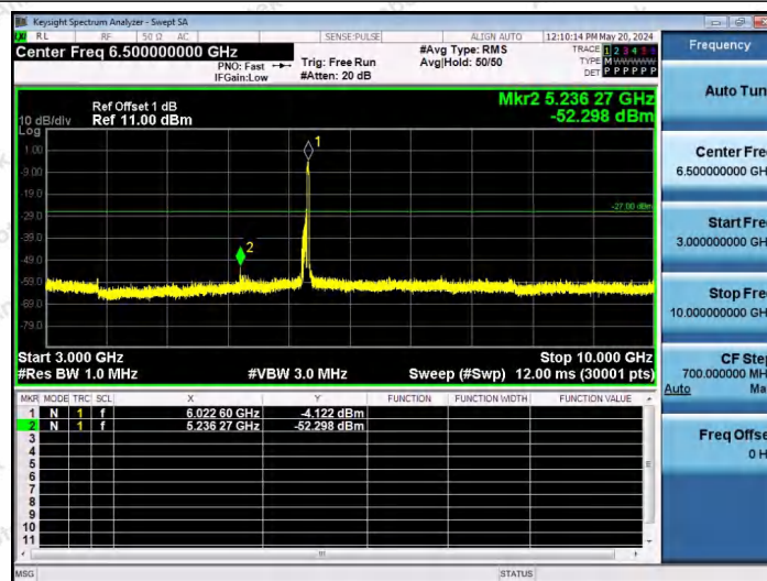
11AX80SISO-Ant1-5985-242Tone-RU64-3000~10000-PASS
