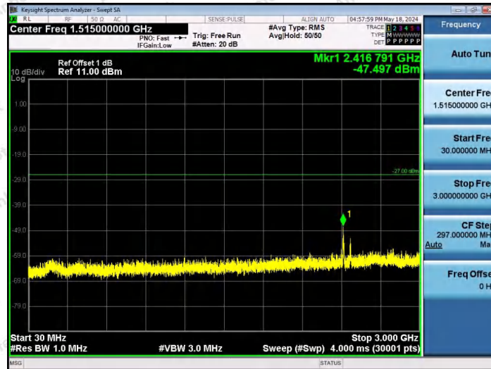
11AX40SISO-Ant1-6885-242Tone-RU61-30~3000-PASS
