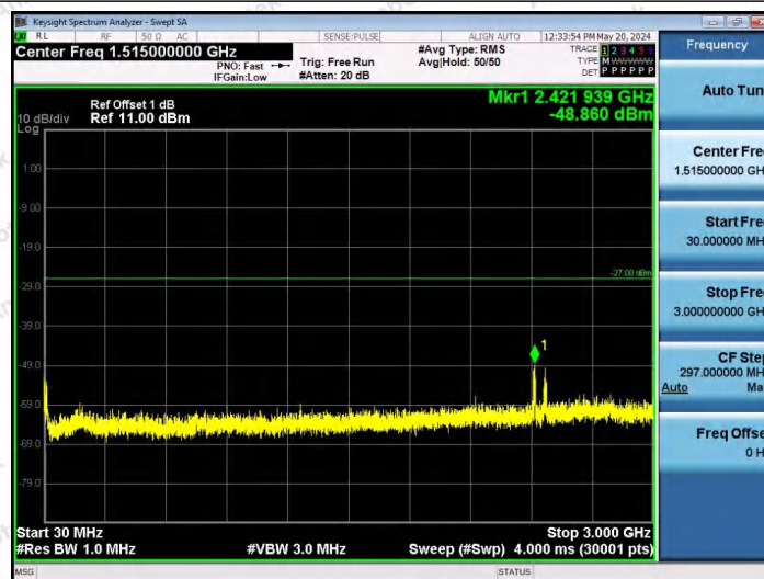
11AX80SISO-Ant1-6145-106Tone-RU60-30~3000-PASS
