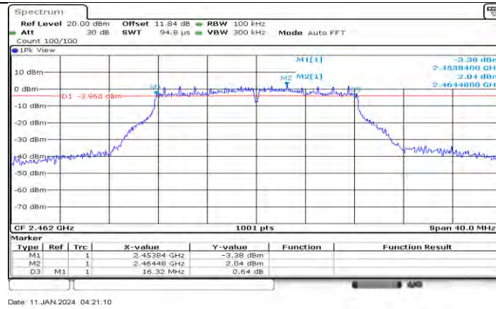
11G-CDD_Ant1_2462
