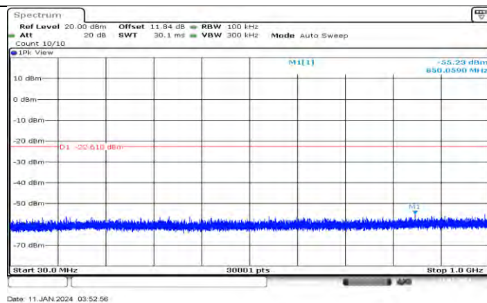
11B-CDD Ant2 2437 30~1000
