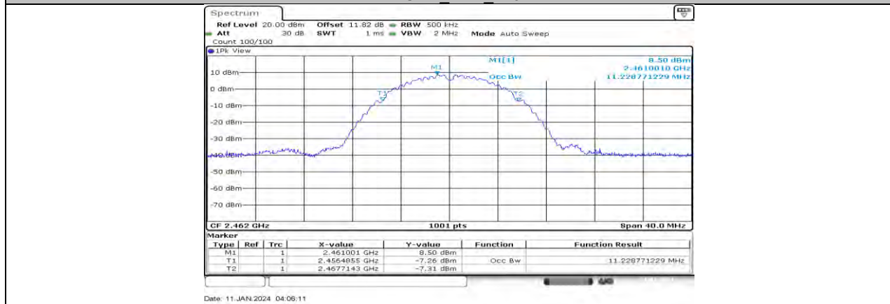
11B-CDD_Ant2_2462
