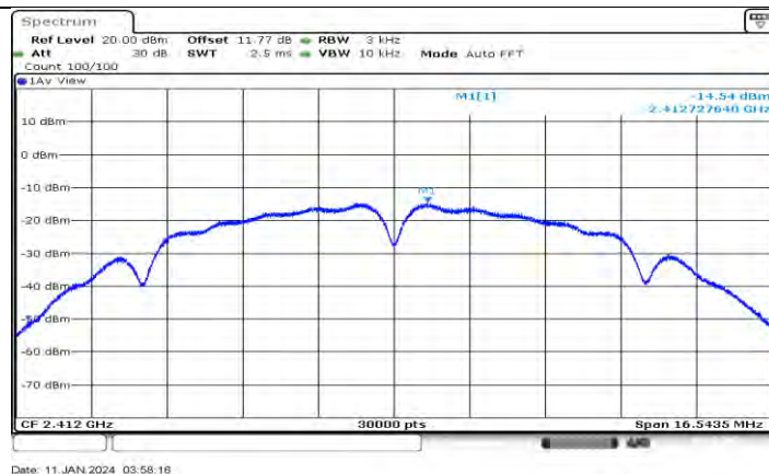
11B-CDD_Ant2_2412
