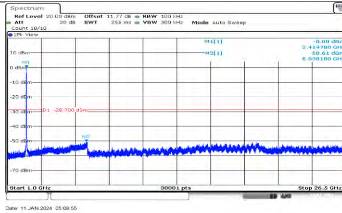
11AX20MIMO_Ant2_2412_1000~26500
