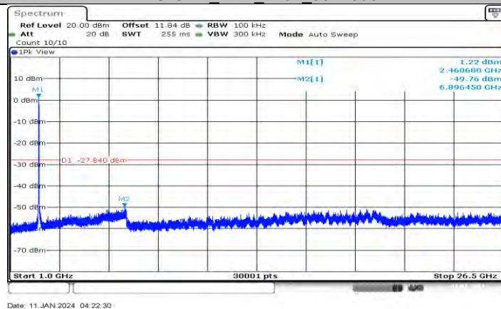
11G-CDD_Ant1_2462_1000~26500
