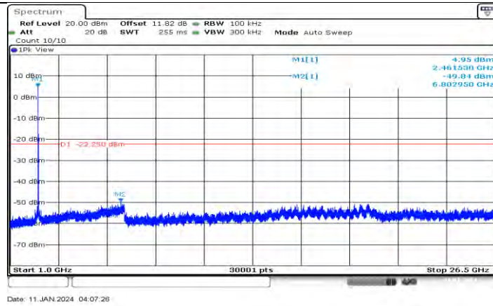
11B-CDD Ant2 2462 1000~26500
