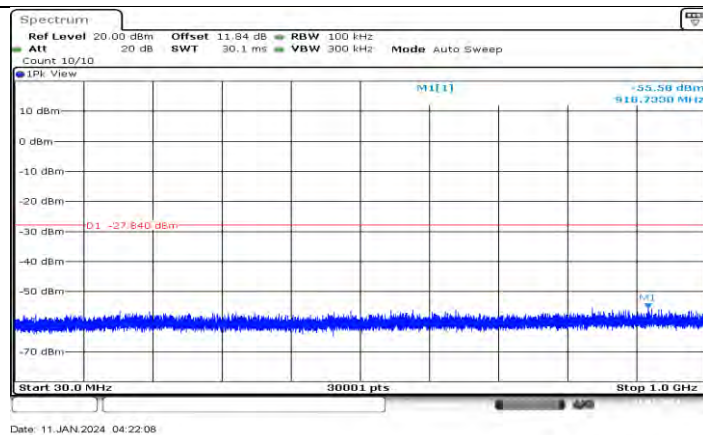
11G-CDD_Ant1_2462_30~1000
