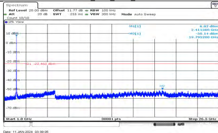
11B-CDD_Ant2_2412_1000~26500
