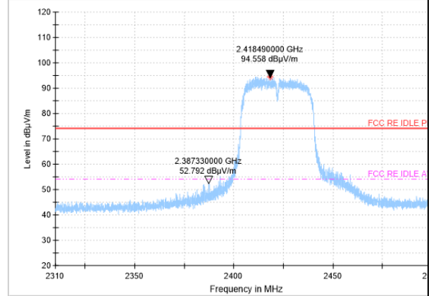
AV detector
