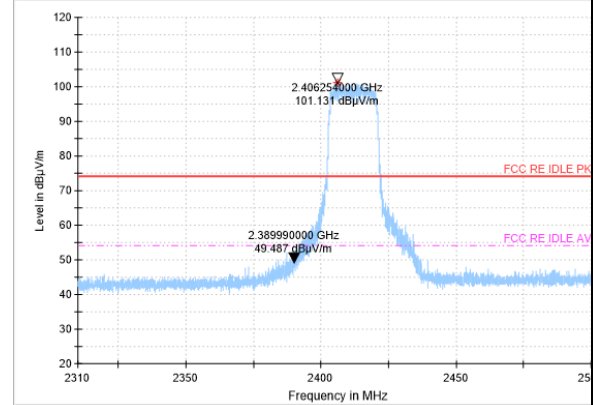
AV detector
