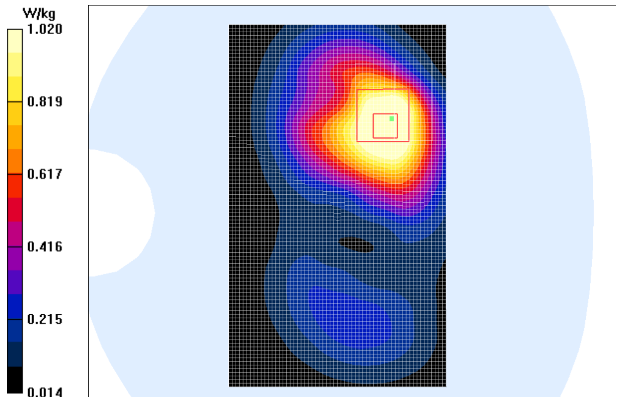
Fig.I.8 WCDMA1900 CH9262
