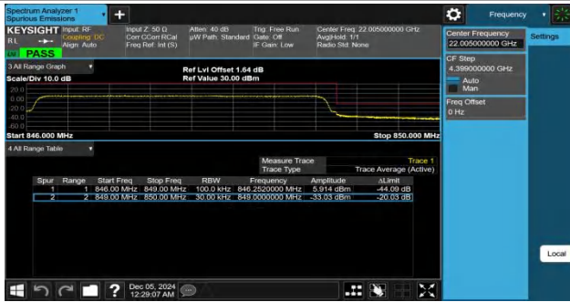
Band26(824-849)-3MHz-QPSK-27025-15RB#0-PASS
