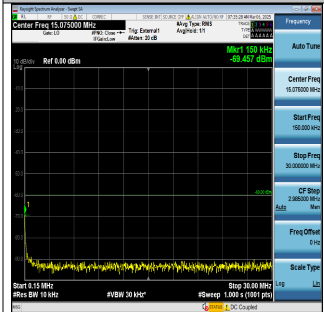
48-48-20MHz-20MHz-QPSK-QPSK-55891-56089-1RB#0-ORB#0-0.15~30MHz-PASS
