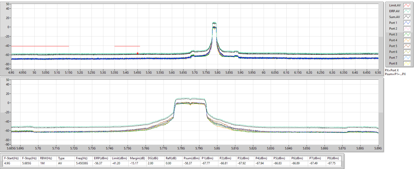
802.11a_Nss1,(6Mbps)_8TX 5785MHz
