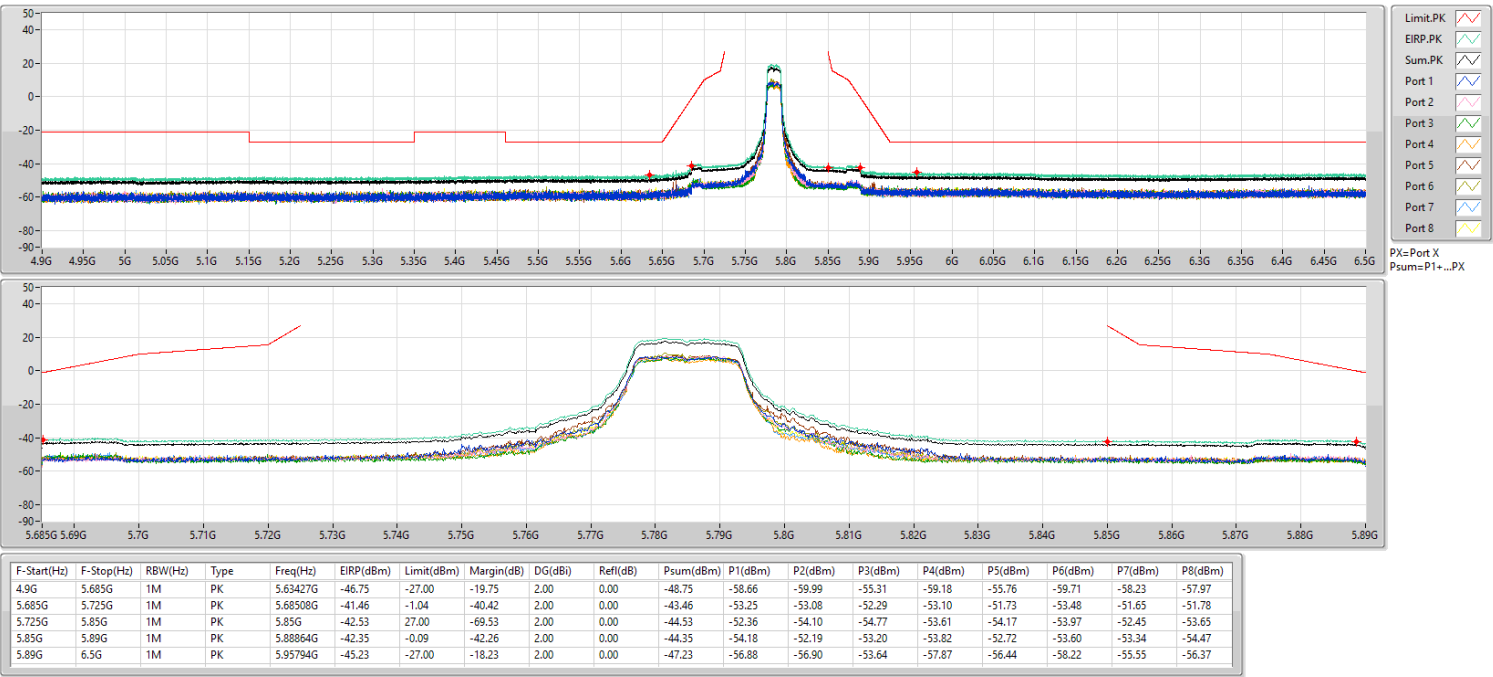
802.11a_Nss1,(6Mbps)_8TX 5785MHz
