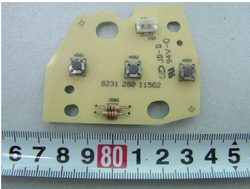
EUT- Fan Control PCB Top View
