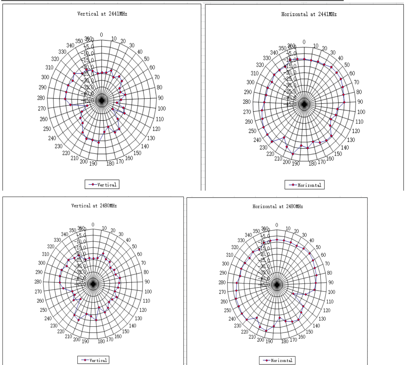
BT Antenna Gain Y
