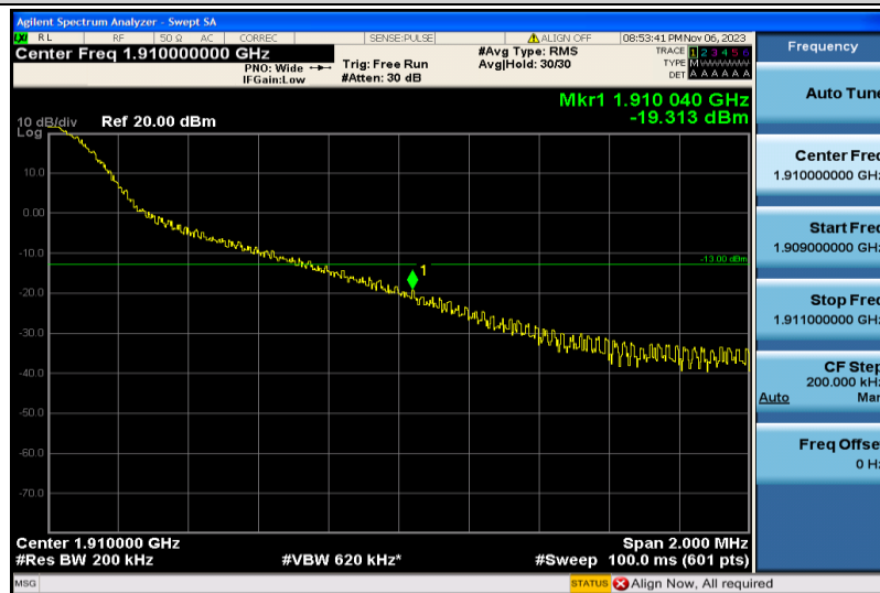
Band2-20MHz-QPSK-19100-1RB#99
