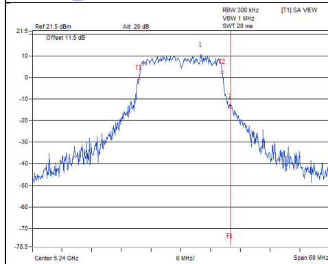
802.11a_Chain 2 / CH48
