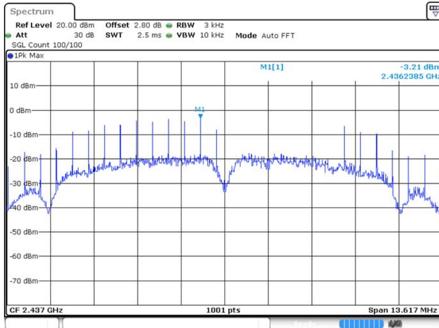
Test_Graph_802.11b_ANT1_2437
