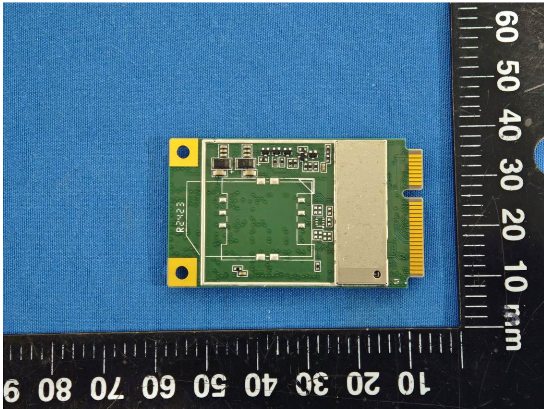
NFC Module
