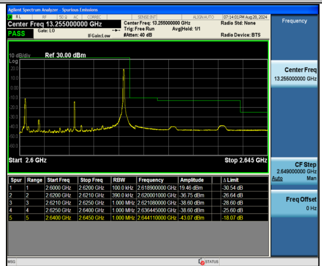
Band38-20MHz-QPSK-38150-1RB#99-PASS
