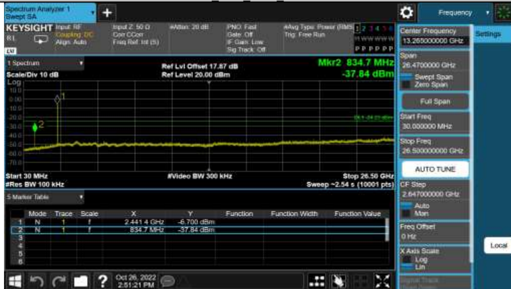
2DH5 Ant1 2441 30~26500
