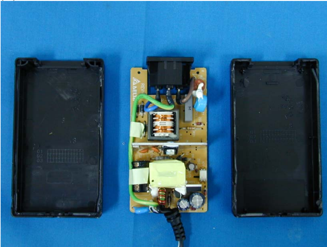
(17) EUT Photo-Mode 2
