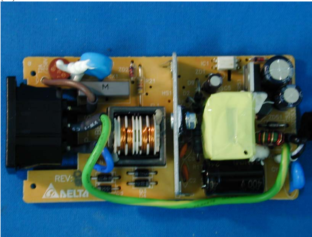
(18) EUT Photo-Mode 2
