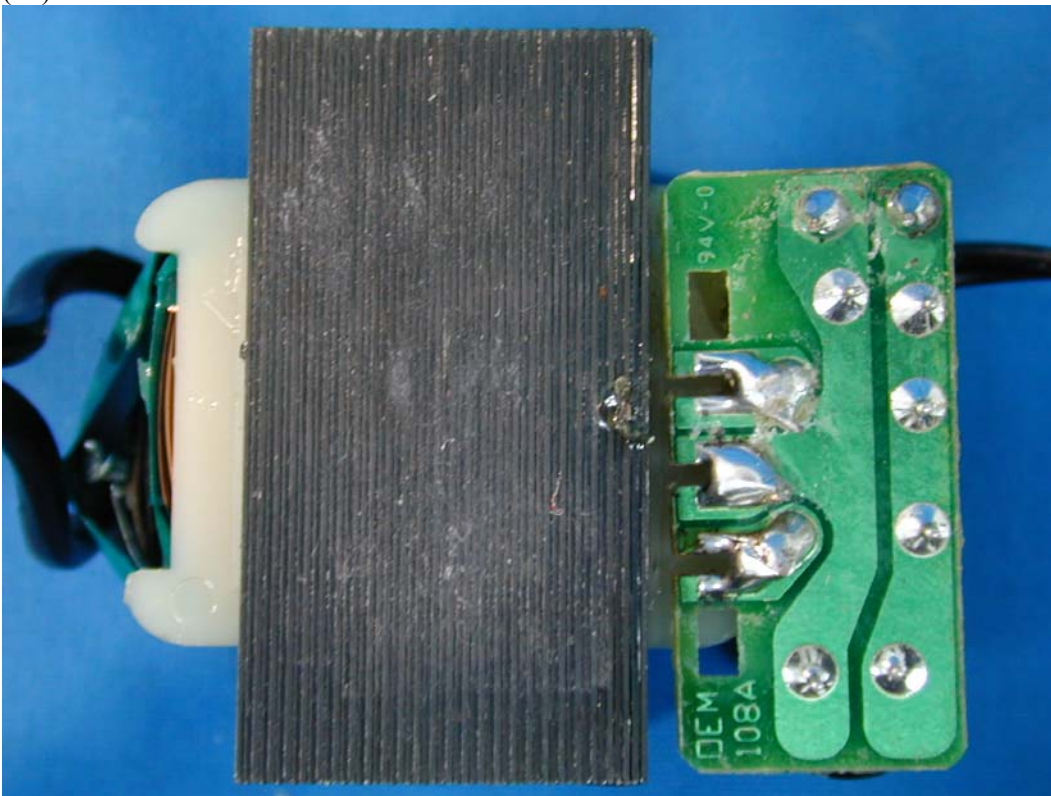
(16) EUT Photo-Mode 1
