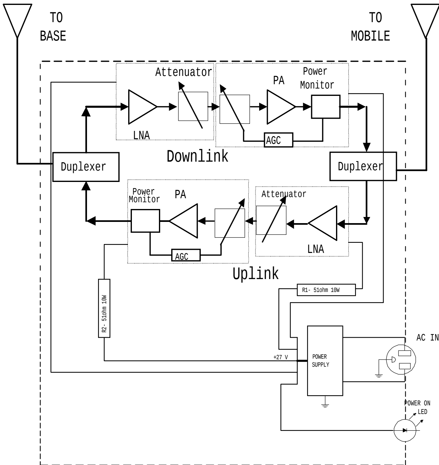
CBDA-ESMR-1W80-A ELECTRICAL SCHEMATICS
