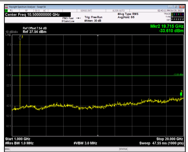
Band2-20MHz-QPSK-18700-1RB#0-Range2:1000~20000MHz
