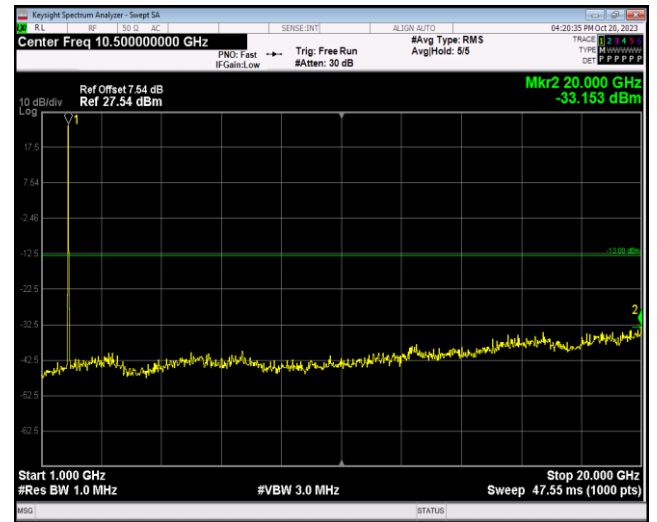
Band2-20MHz-QPSK-18900-1RB#0-Range2:1000~20000MHz
