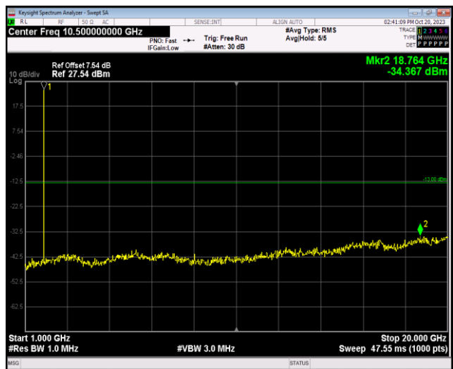
Band2-1.4MHz-QPSK-18900-1RB#0-Range2:1000~2 0000MHz
