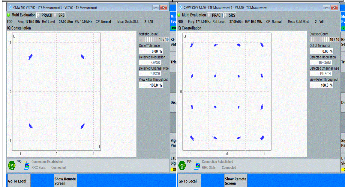
Band4-10MHz-QPSK-20000-50RB#0-PASS
