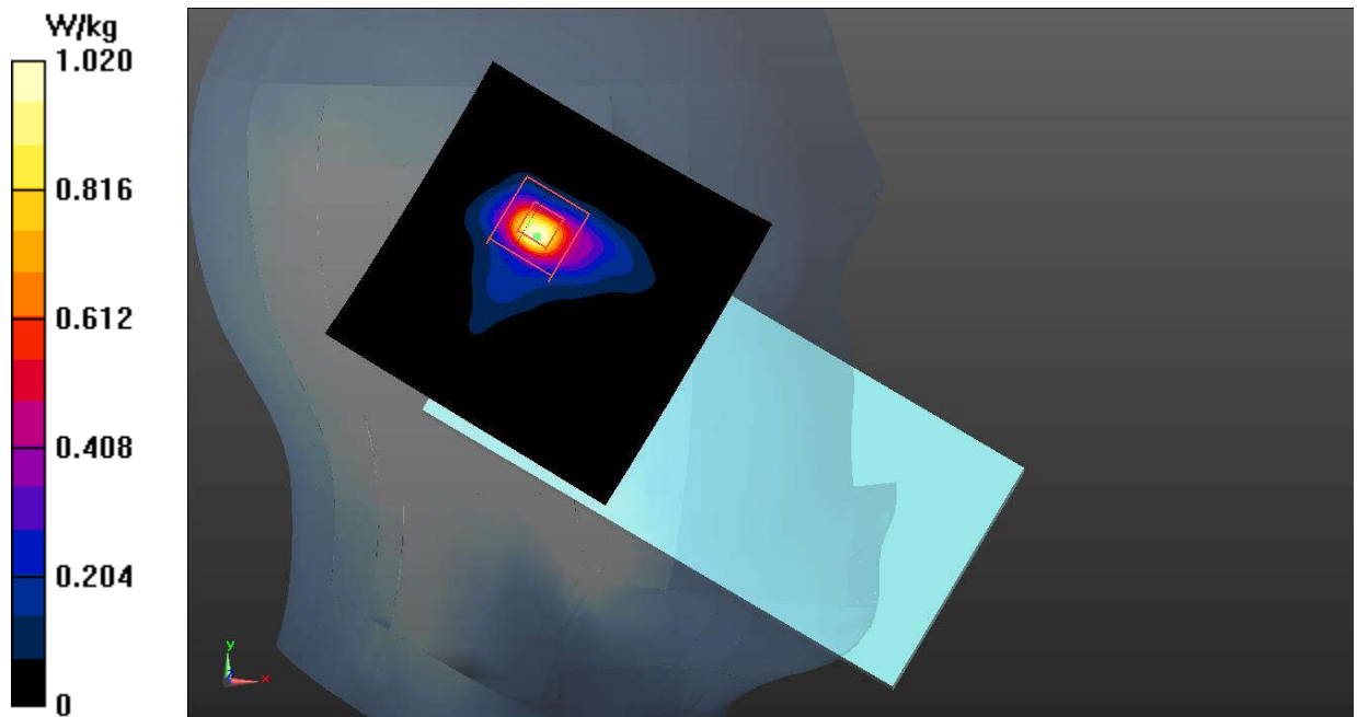
Fig.40 WLAN 5G
