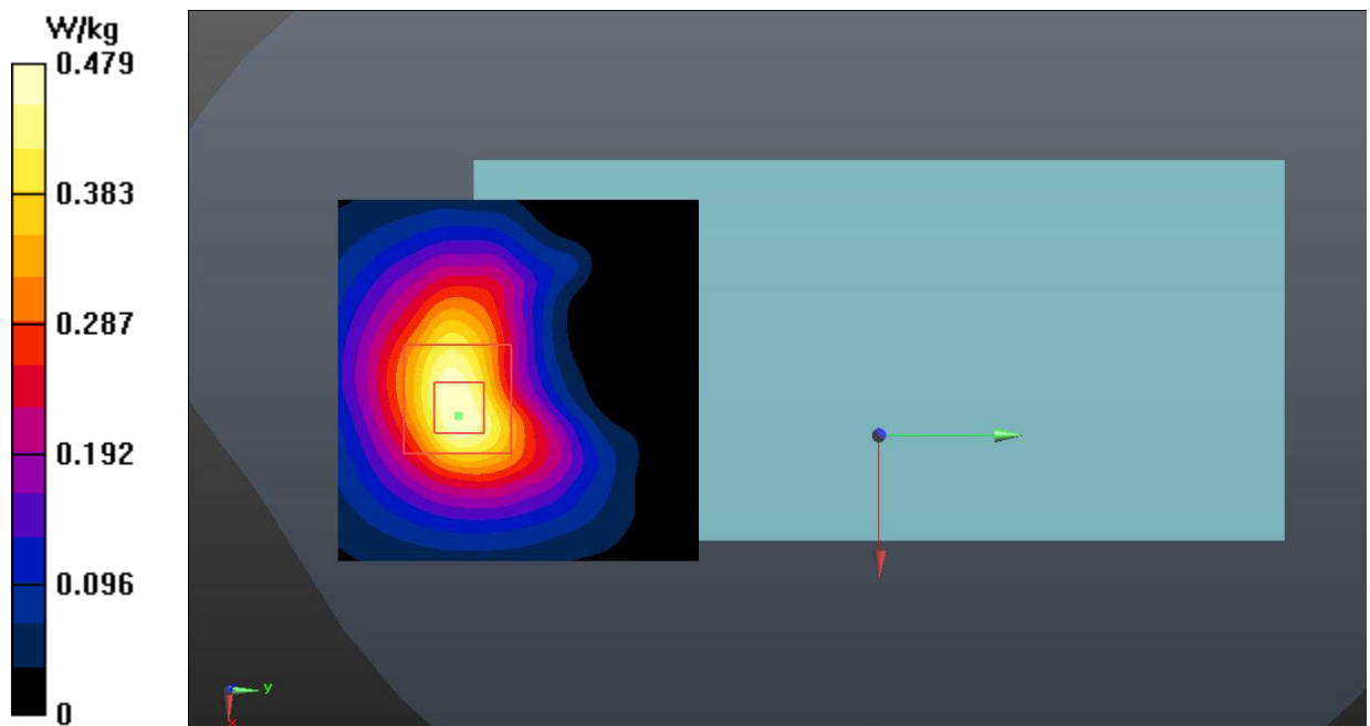
Fig.41 WLAN 5G
