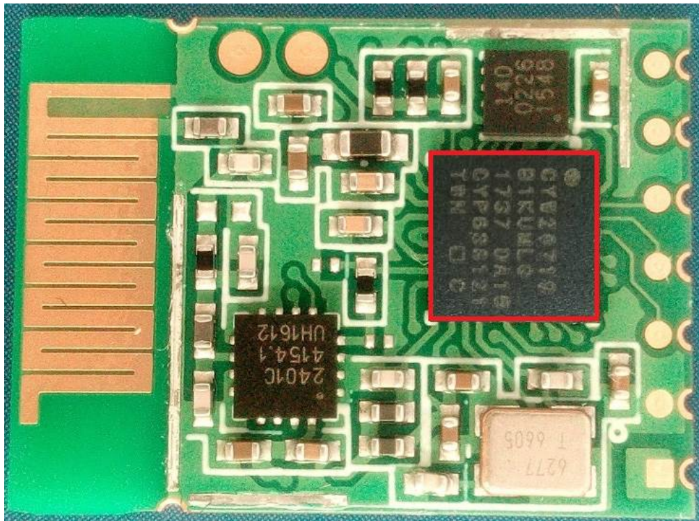
(4) EUT Photo ( CYBLE-413149-01 )
