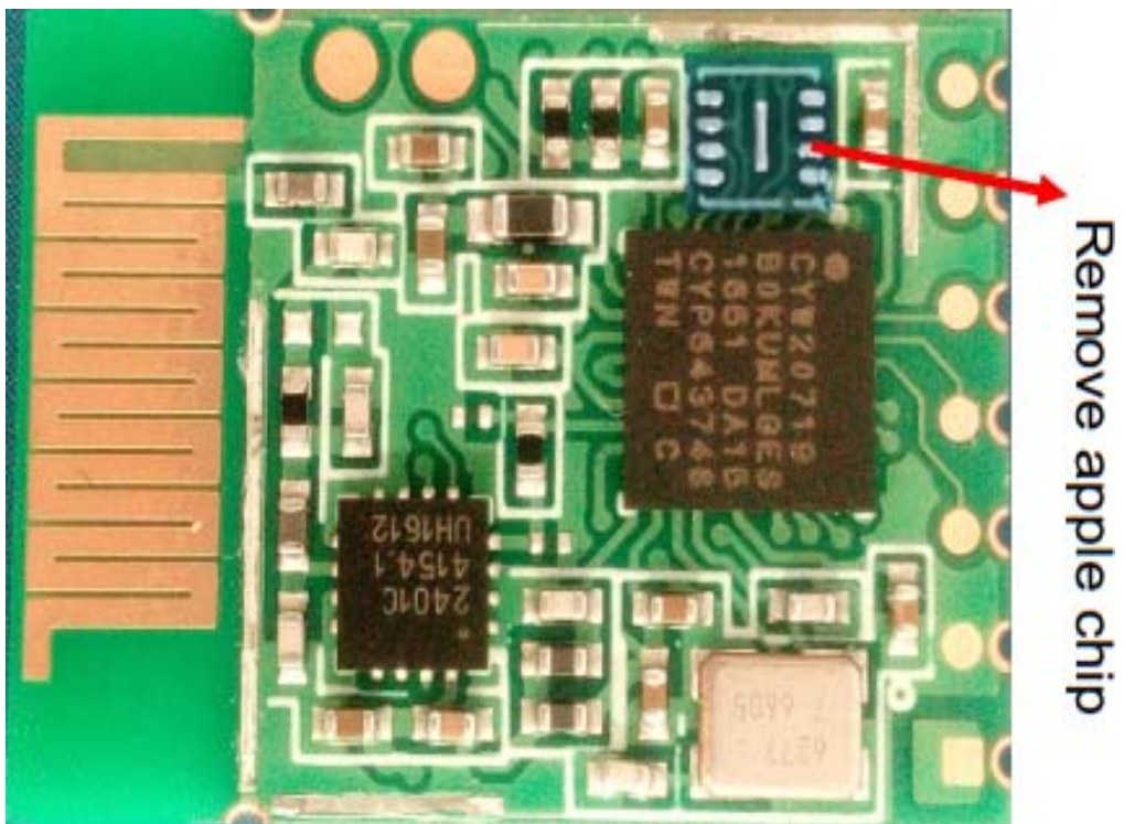
(4) EUT Photo ( CYBLE-413149-01 )
