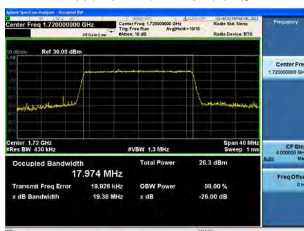
Band66 / 20MHz / Low CH / 64QAM
