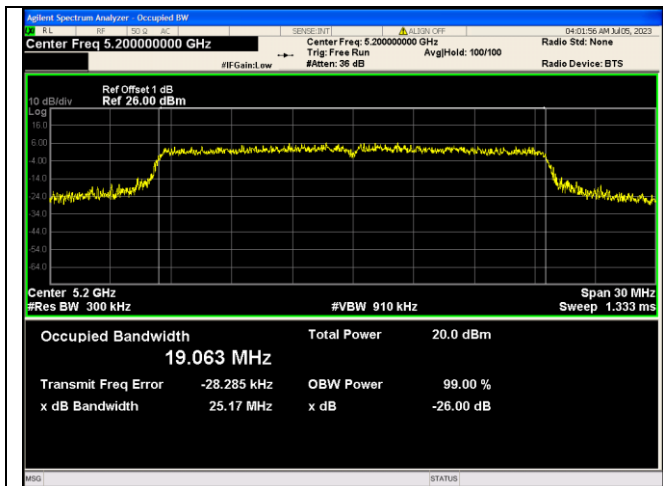
IEEE 802.11ax_Channel 40_20MHz_Antenna 0_RU&amp;Index 242RU61
