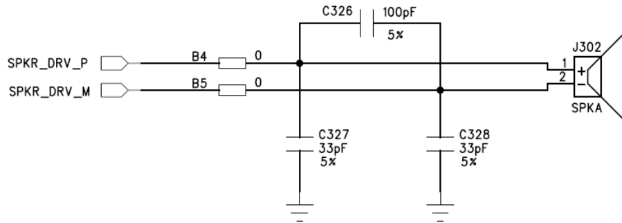
图 4.24: 用内部音频功放推荐电路
