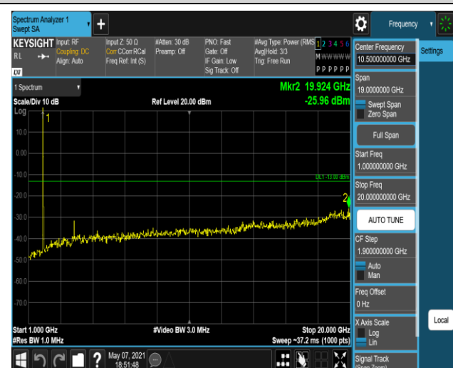
Band2-20MHz-QPSK-18900:1000~20000MHz
