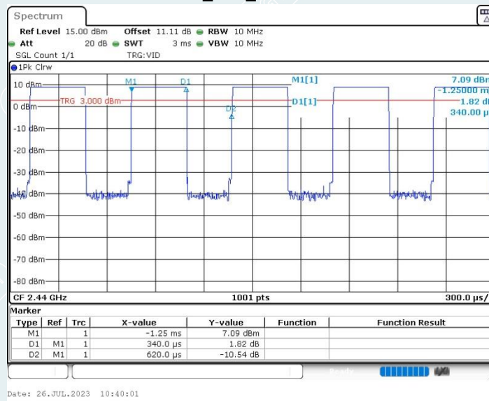
BLE_1M_2440MHz
