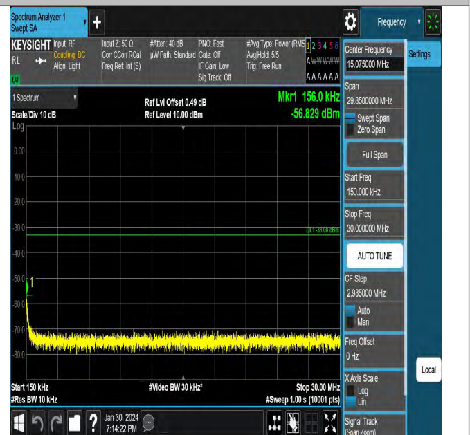
GSM1900-810-0-0.15~30MHz-PASS
