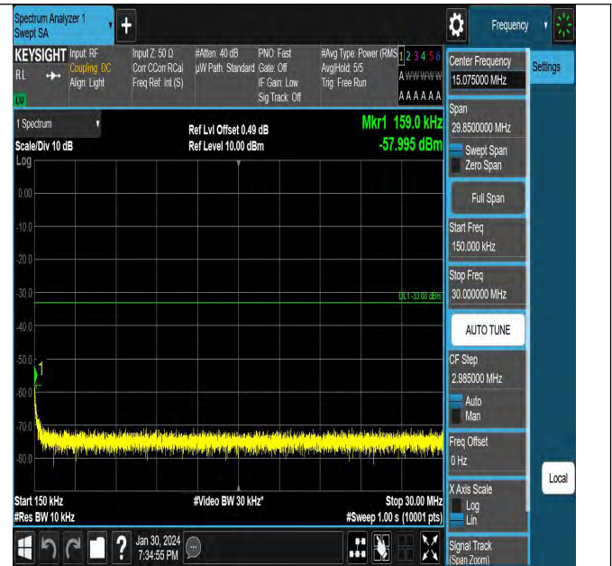
EGPRS1900-810-2-0.15~30MHz-PASS
