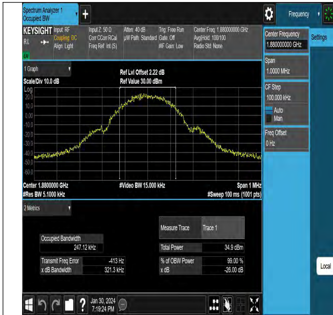
GPRS1900-661-0-PASS
