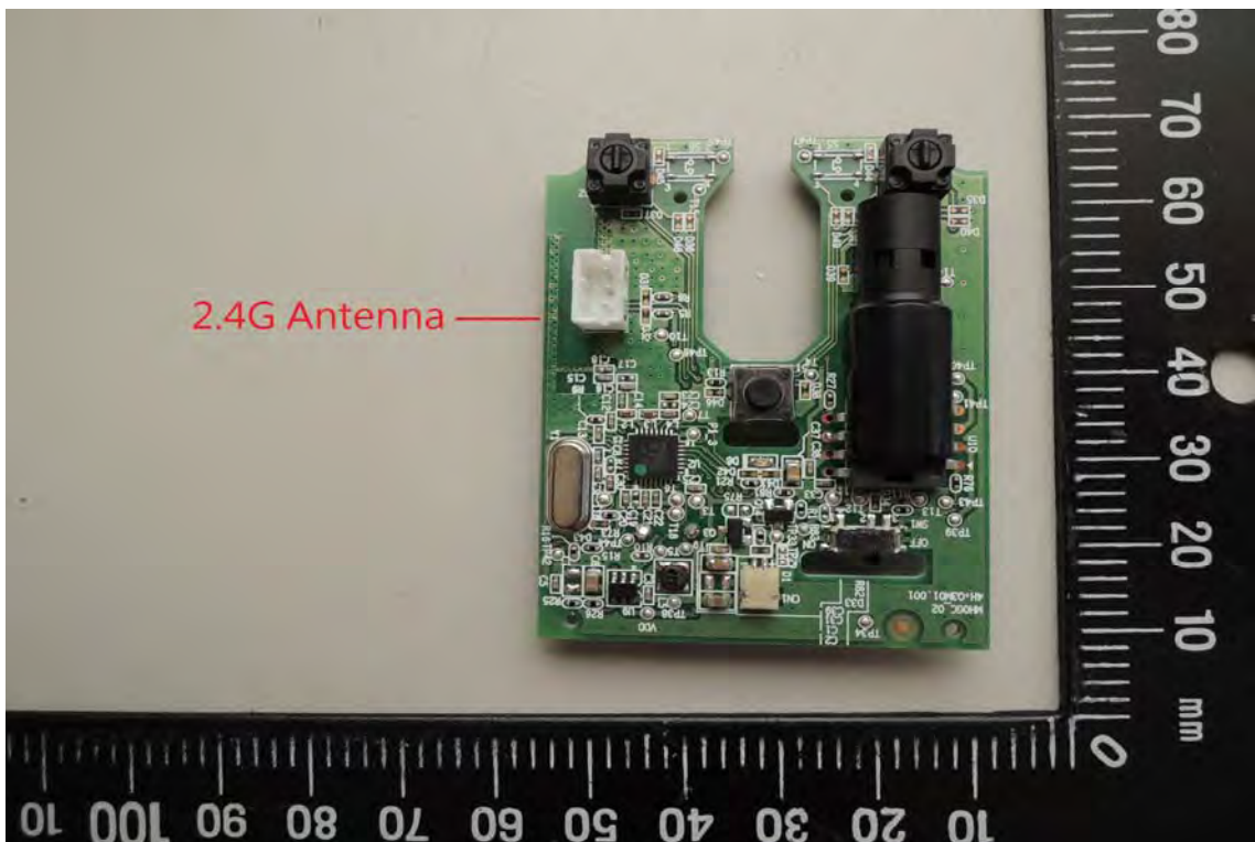
2.4G Antenna
