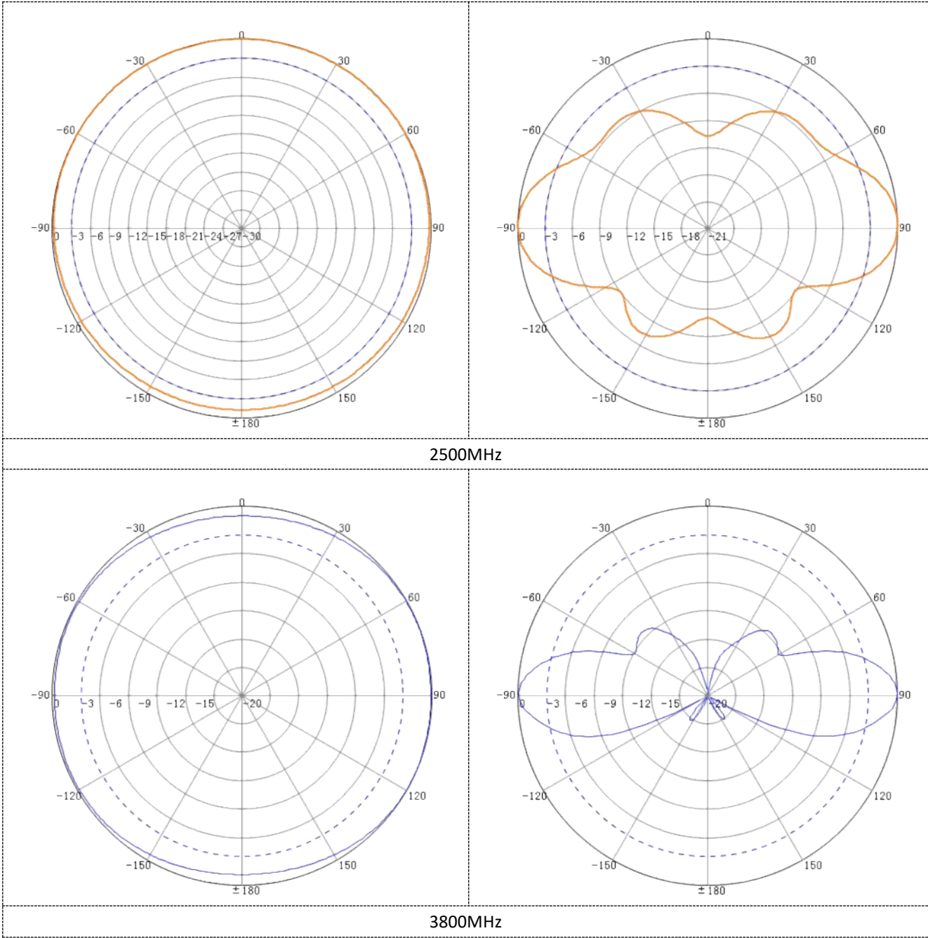
H-Pattern
