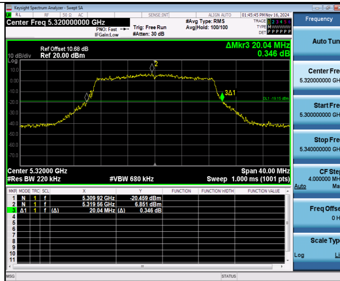
11AC20MIMO_Ant W1_5320
