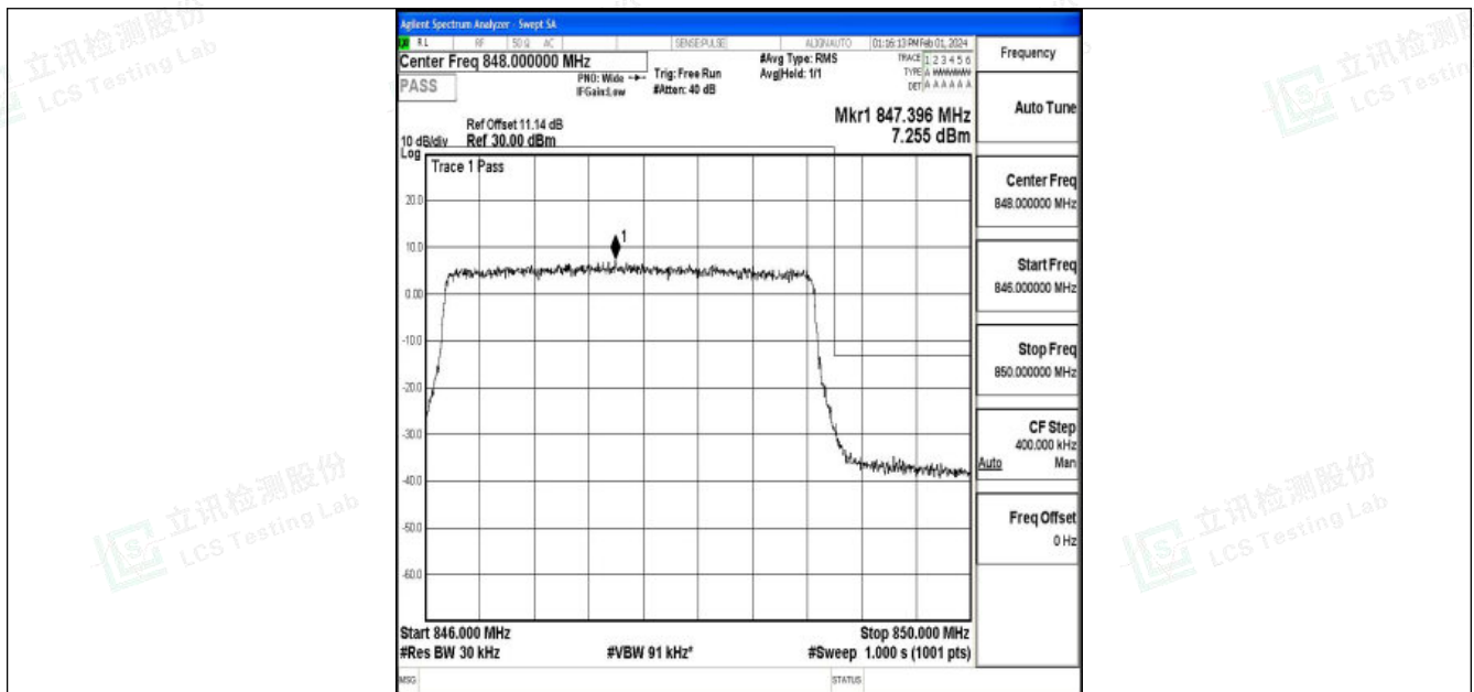
Band5_3MHz_16QAM_20635_15RB#0
