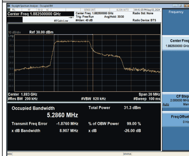
Band25-10MHz-16QAM-26365-27RB#0-PASS
