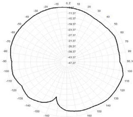
923.0MHz Total(E1-XZ), Max= -7.37dBi
