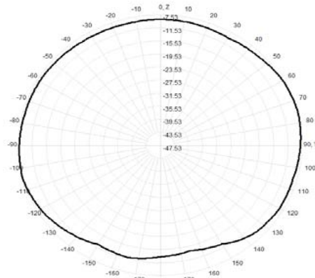
921.0MHz Total(E2-YZ), Max= -7.54dBi
