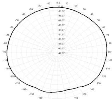
923.0MHz Total(E2-YZ), Max= -7.54dBi
