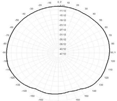
930.0MHz Total(E2-YZ), Max= -7.20dBi
