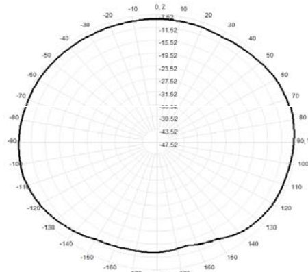
922.0MHz Total(E2-YZ), Max= -7.55dBi
