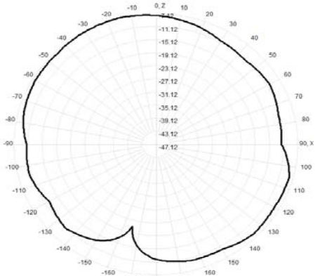
930.0MHz Total(E1-XZ), Max= -7.12dBi
